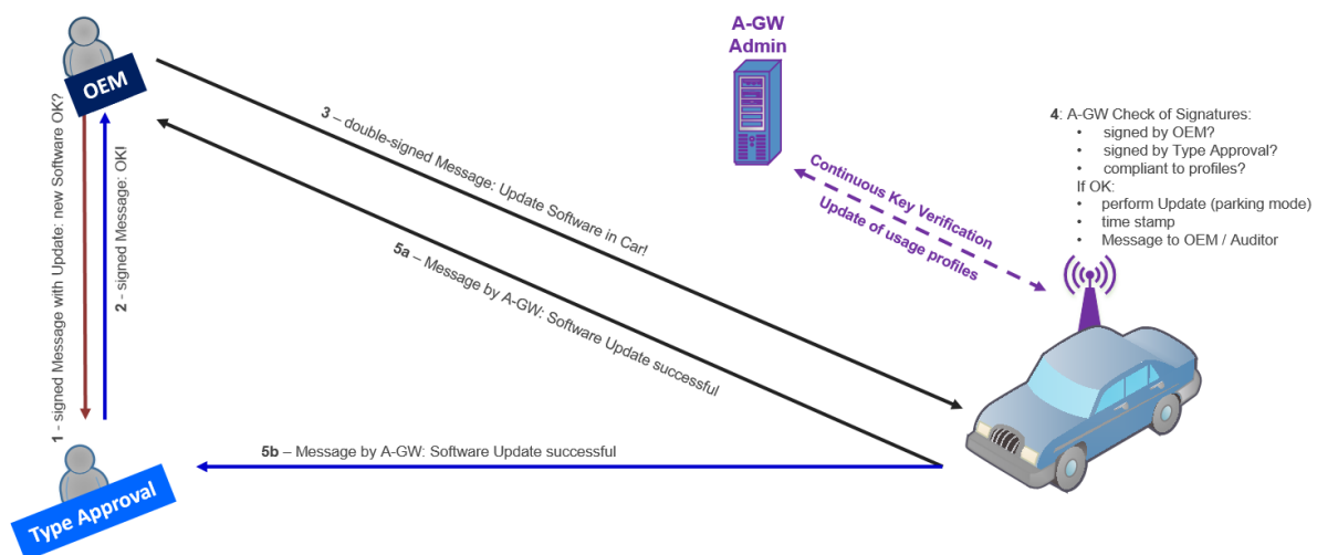
Abbildung 18: Software Update durch einen OEM (vereinfachtes Beispiel)
