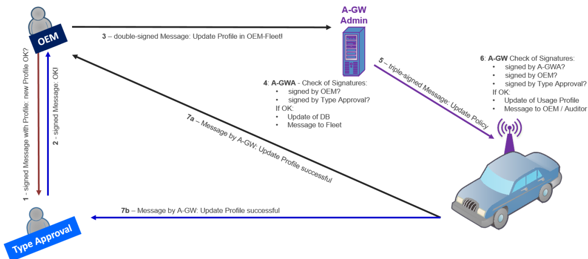
Abbildung 17: Update eines OEM Usage-Profiles (vereinfachtes Beispiel)
