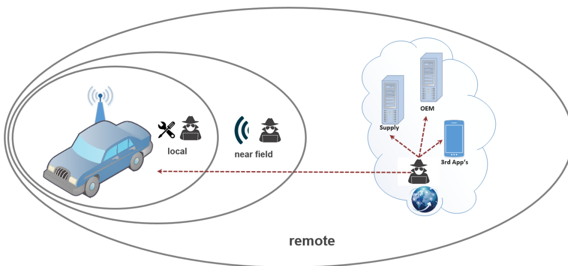
Abbildung 8: Mögliche Angriffsvektoren
